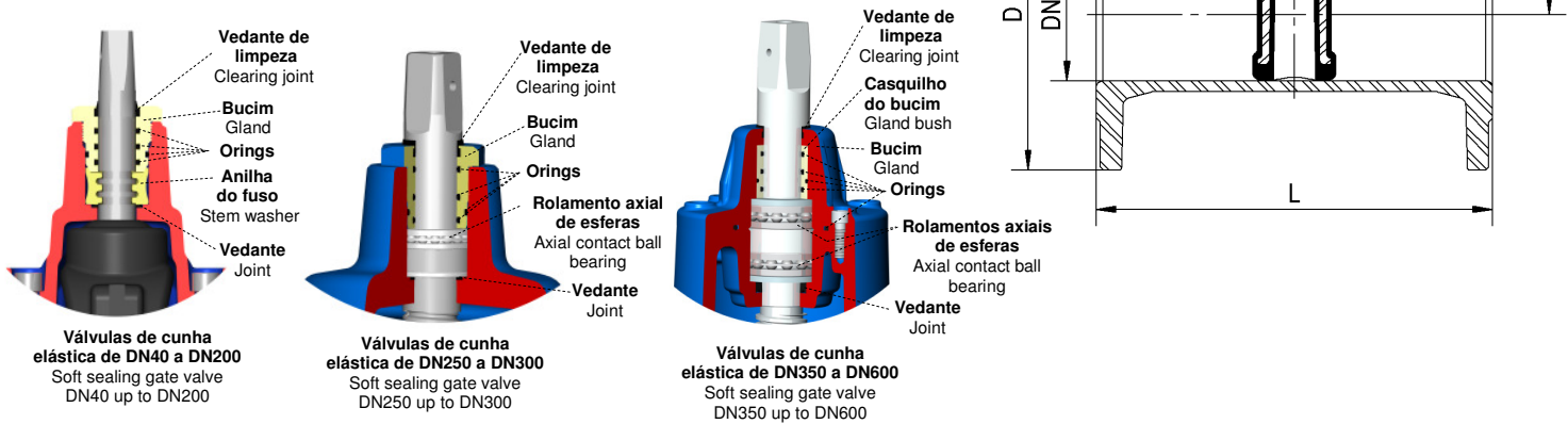
Pormenor da vedação do Fuso Stem sealing detail
